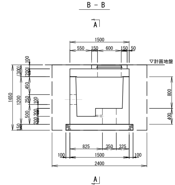
取水ピット(ポンプ室)図 S=1:60
