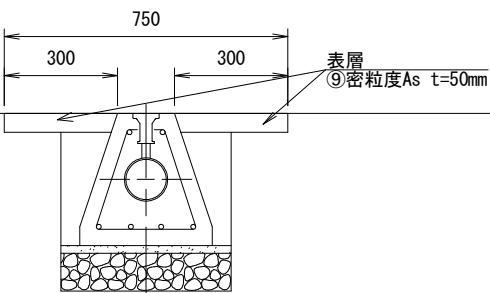
二次施工標準断面図
