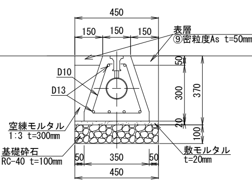
一次施工標準断面図
