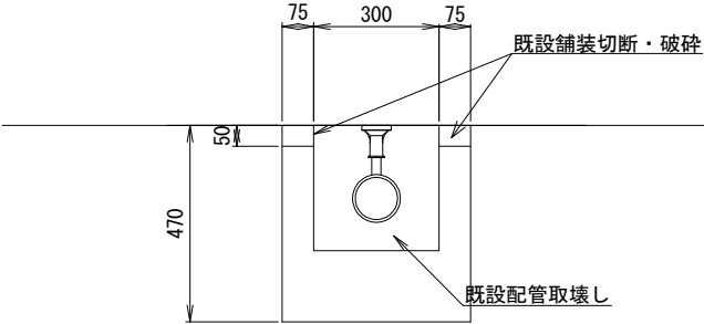
現況断面図
