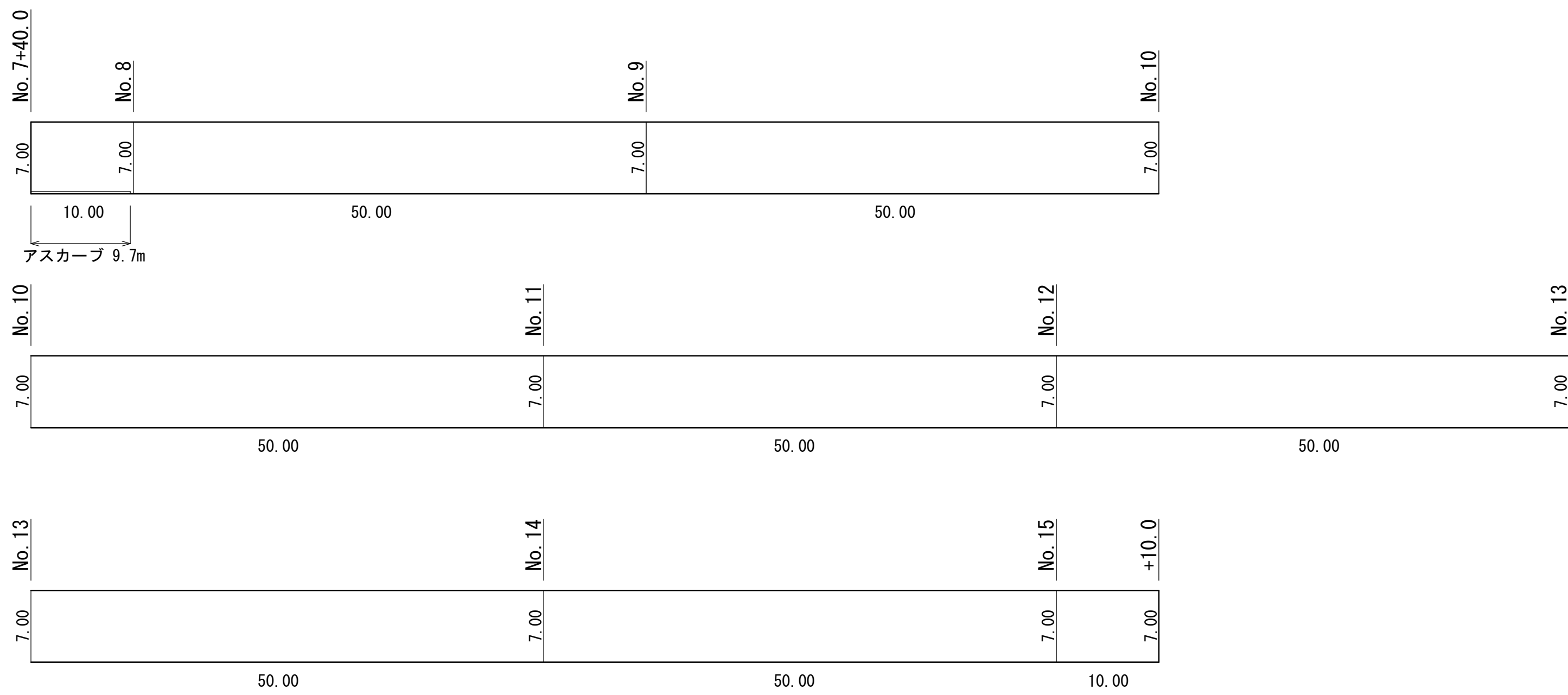
アスカーブ断面図 1:10
