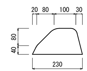
アスカーブ断面図 1:10
