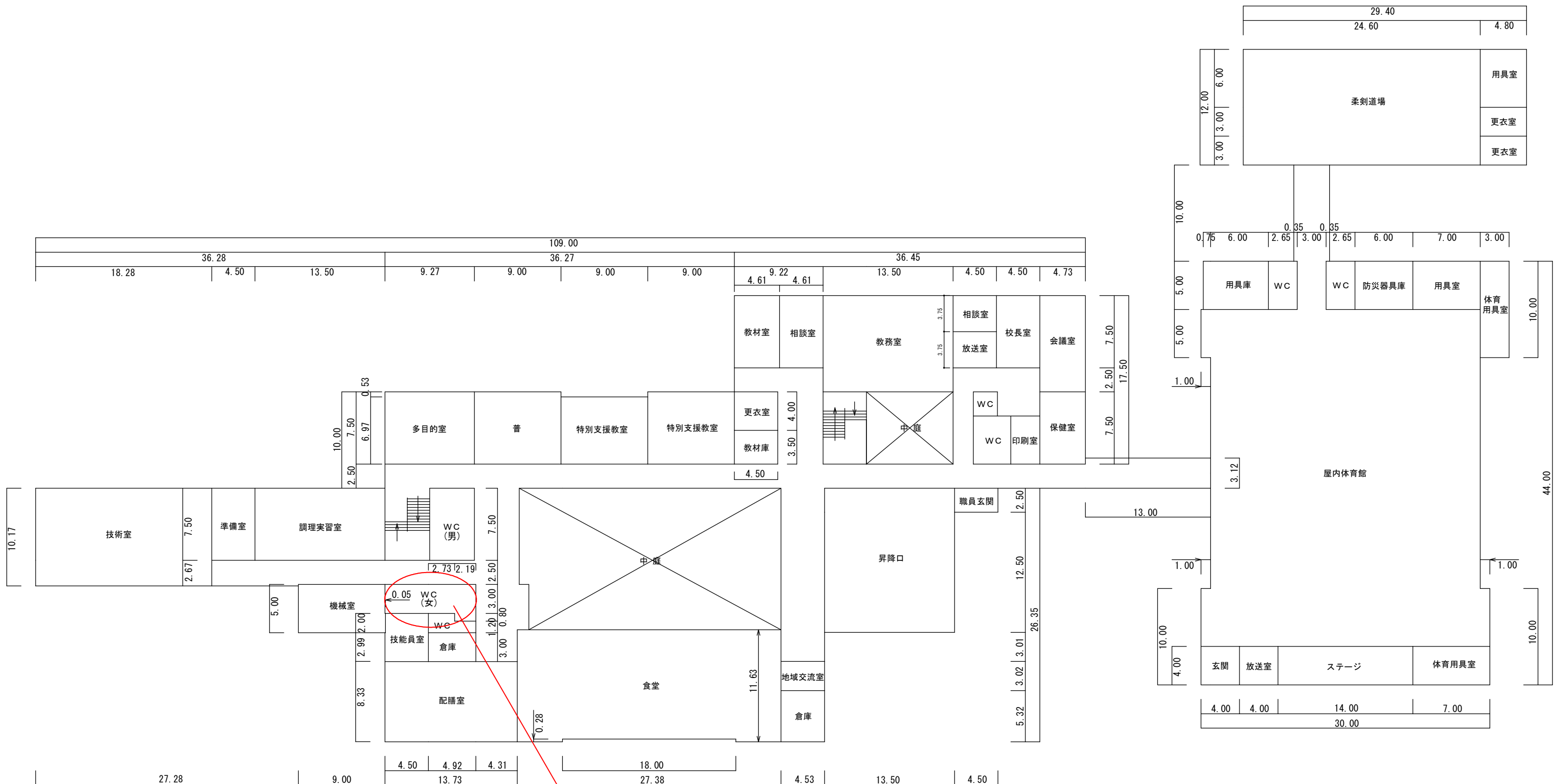
【1F女子トイレ配置図】
