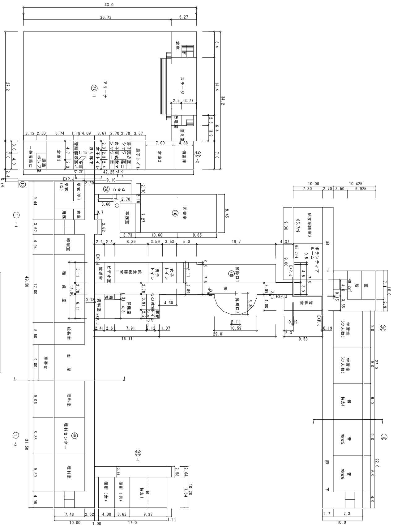
1 階平面図
