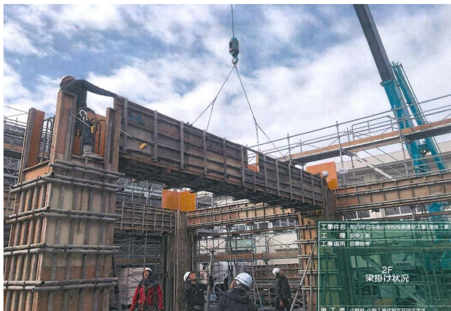
▲図書館棟躯体梁型枠組立
