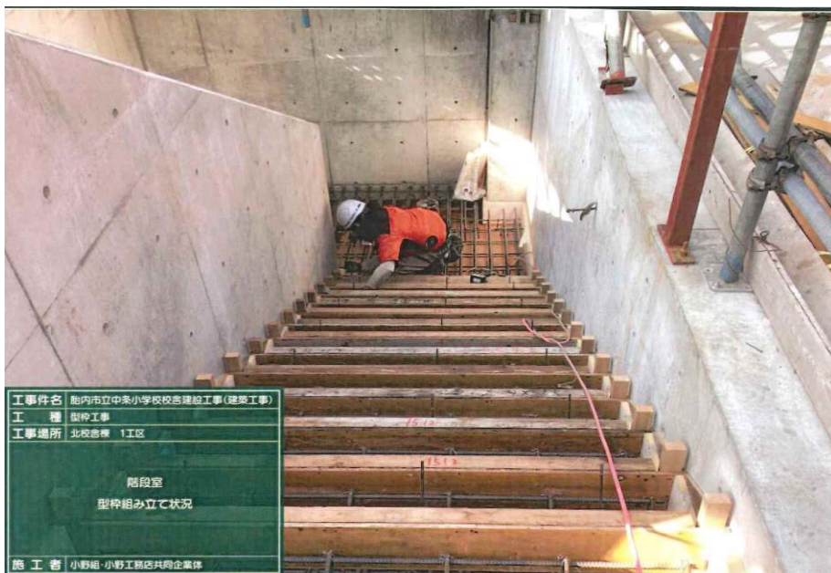
▲北校舎階段型枠
